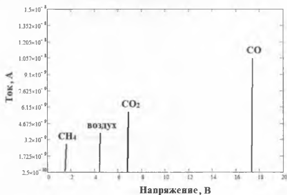
Рис. 2. Зависимости тока разряда от напряжения для различных газов
