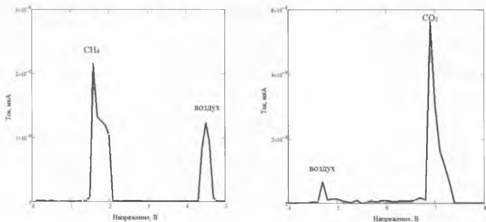
Рис. 1. Вольтамперные характеристики измеренные для CH_4 +воздух (а) и CO_2 +воздух (б)
