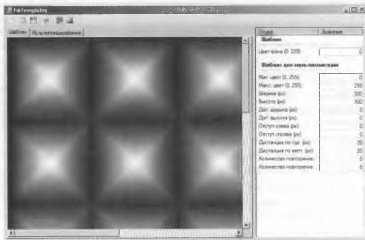
Рис. 1. Интерфейс программы
