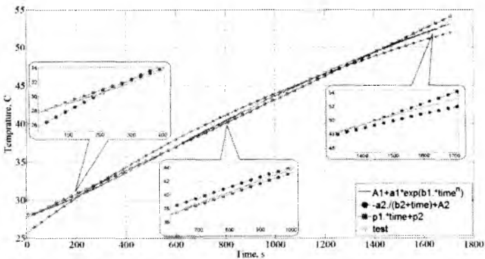
Рис. 2. Сравнительный анализ экспериментальных и расчетных характеристик (с экспериментальной кривой)
