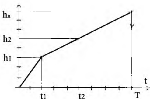
Рис. 1. Тепловая схема прогнозирования ресурса силового оборудования
