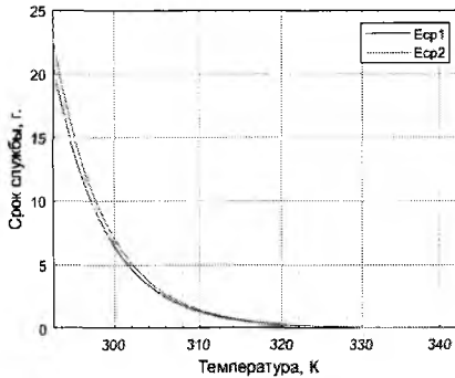
Рис. 6. Зависимость срока службы изоляции от температуры
