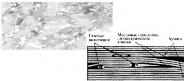
Рис. 2. а – поверхность бумаги, б – структура фрагментов бумажно-масляной изоляции
