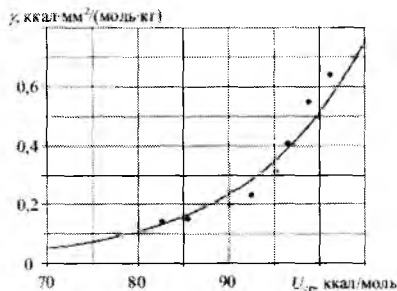
Рис. 5. Зависимость коэффициента \gamma от средней энергии мономерного звена для полимерных материалов
