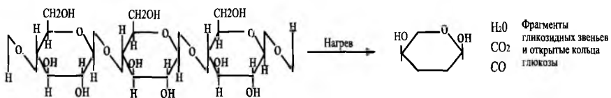
Рис. 3. Процессы деградации целлюлозы и их основные продукты
