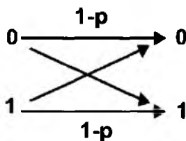
Рис. 3. Симметрический двоичный канал
