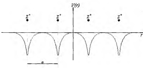
Рис. 5. Качественный вид потенциала цепочки ионов
