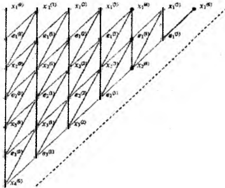
Рис. 1. Граф первой схемы QD-алгоритма Рутисхаузера
