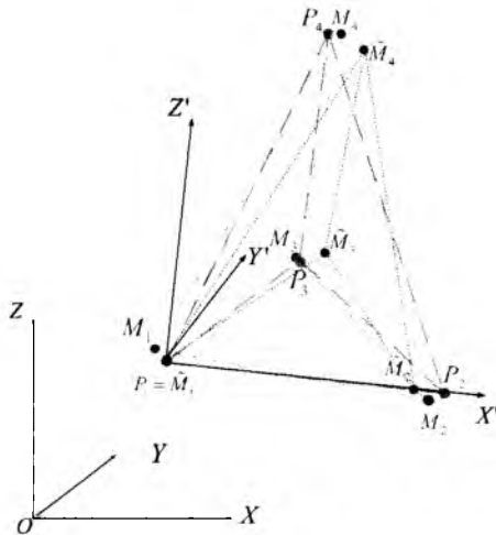
Рис. 3. Определение начального положения тетраэдра, соответствующего начальному приближению для решения оптимизационной задачи (7), по исходному набору точек-оценок
