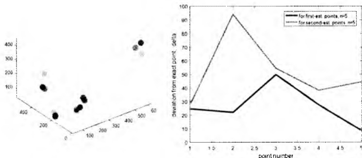
Рис. 8. Результаты уточнения координат для 5 БЛА при невыполнении достаточных условий (19) \sigma_1=29,8 м, \sigma_2=56,7 м
