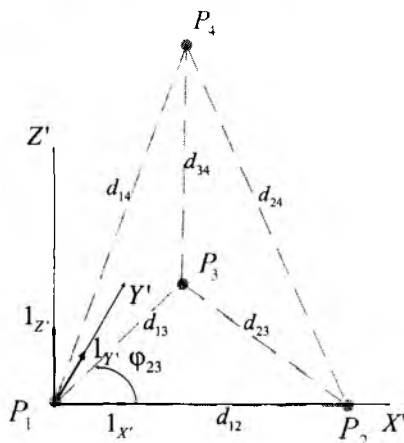
Рис. 2. Локальная система координат подвижного тетраэдра
