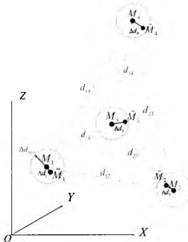
Рис. 1. Истинные и оценочные положения четырех БЛА в пространстве глобальной системы координат OXYZ
