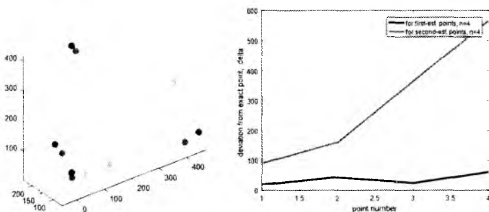
Рис. 7. Результаты уточнения координат для 4 БЛА при невыполнении достаточных условий (19) \sigma_1=51,0 м, \sigma_2=87,3 м
