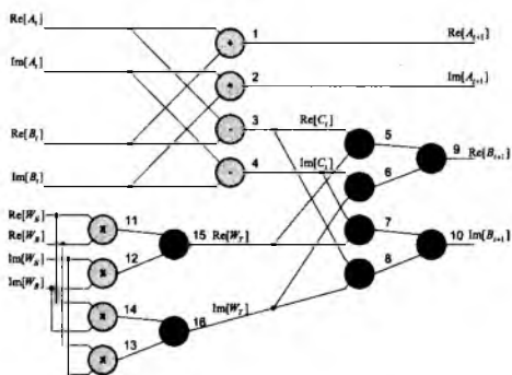
а) Структура из 2-х базовых подграфов
