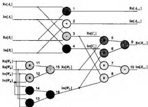
в) Структура из 4-х базовых подграфов
