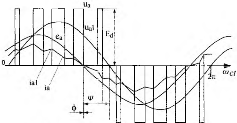
Рис. 3. Осциллограмма напряжений и токов
