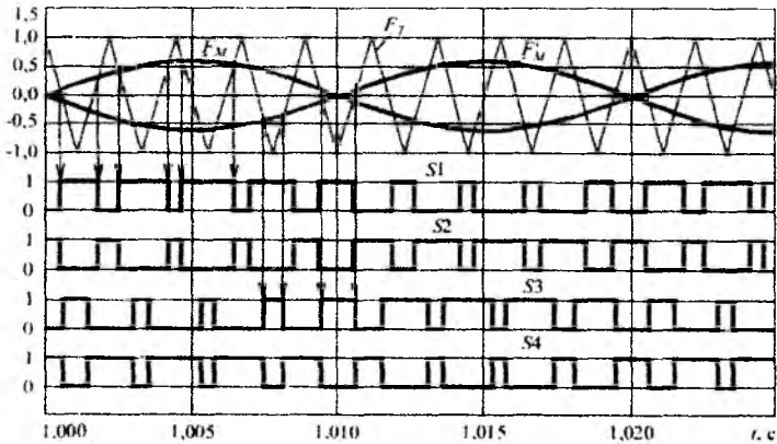
Рис. 4. Получение ШИМ-сигналов управления транзисторами инвертора
