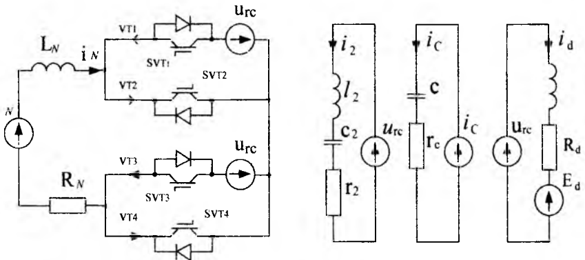
Рис. 2. Разделение схемы с преобразователем 4QS на подсхемы
