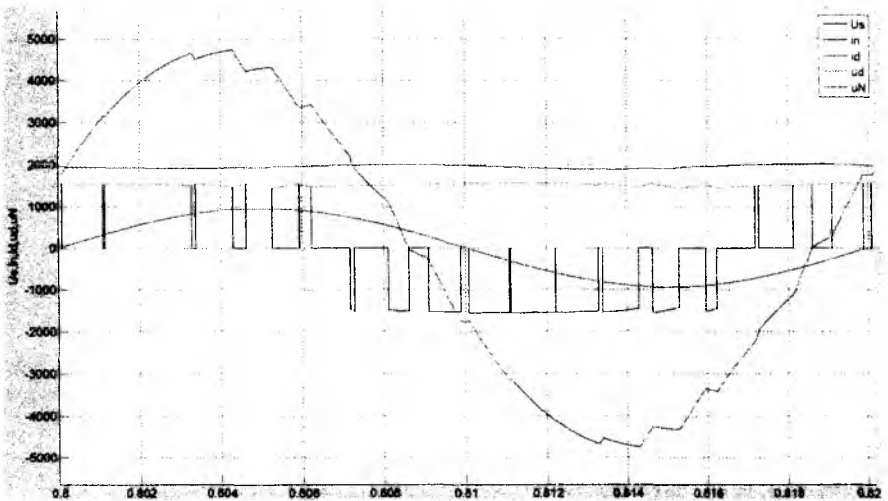
Рис. 7. Моделирование передачи энергии в цепь постоянного напряжения ( \psi = \pi/3,26 )
