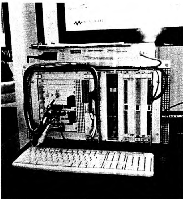
Система функциональ- ного тестиро- вания TS-8989 (слева); фемто/пикоам- перметр B2980A (справа)
