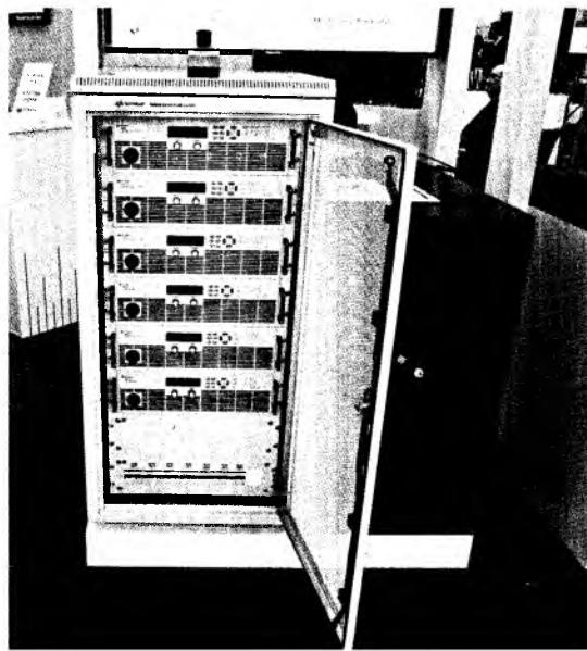
Комплексный источник питания мощностью 90 кВт
