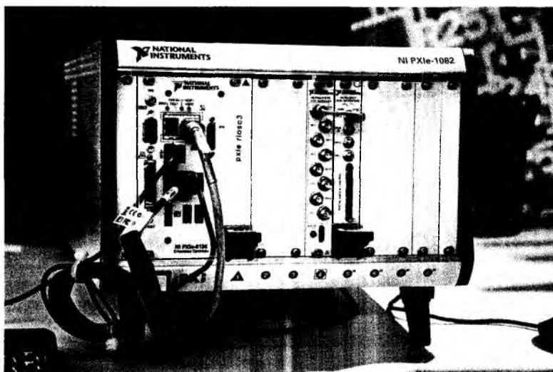
Шасси PXI с установленным осциллографом PXIe-5171R
